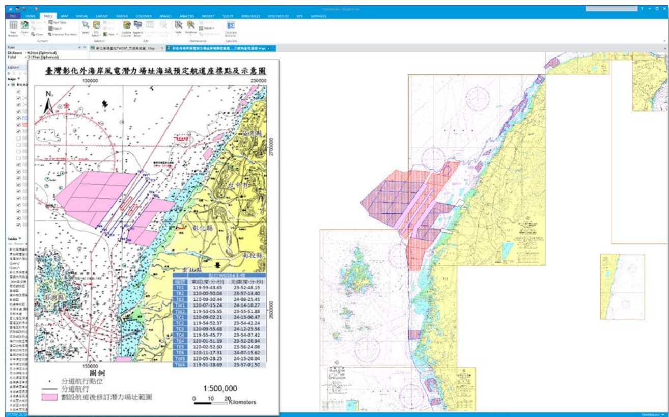
圖 5 因航道管制（左），致使彰濱外海原規劃風場範圍縮小近半（右，橙色部分取消開發）
