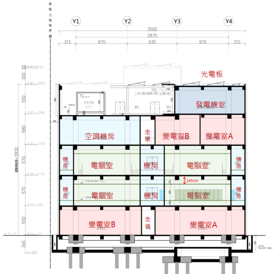
圖 11 空間剖面圖
