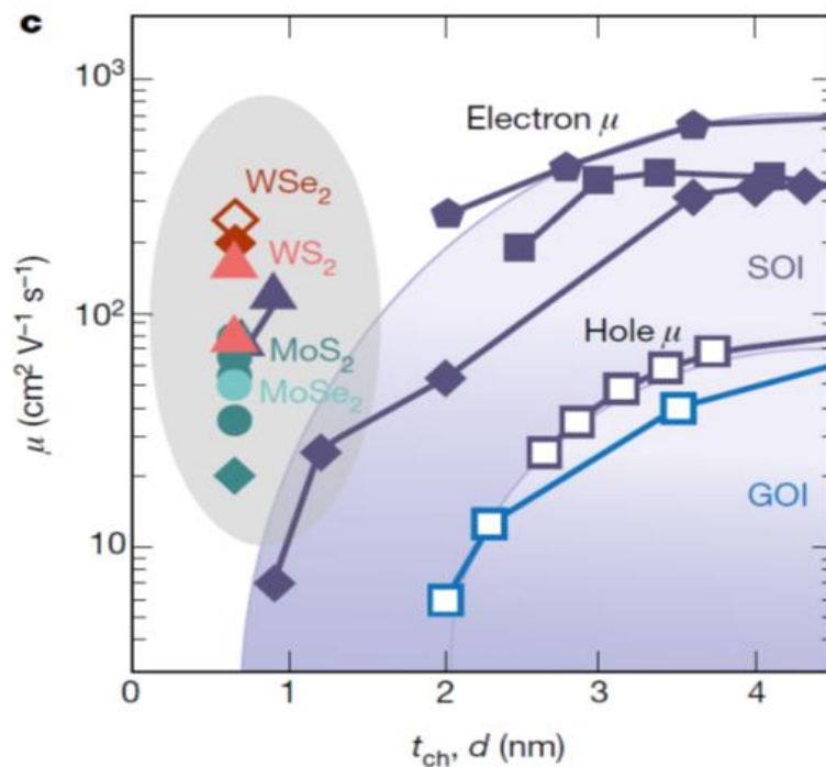
圖 1、傳統半導體與二維半導體中載子遷移率隨著通道層厚度的變化。[ Nature 573, 507-518 (2019)]
