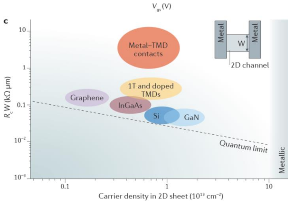
圖 2、各類通道層材料的金屬接觸電阻與通道載子濃度的關係圖。 [ Nat. Rev. Mater. 1, 16052 (2016)]
