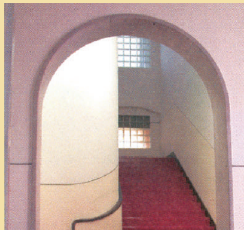
一般建築樓梯為利抗震都設在角落，而行政院樓梯則設在四邊的中段地區，採用SRC (Steel Reinforce Concrete) 鋼骨鋼筋混凝土，具有很好的耐震性。
