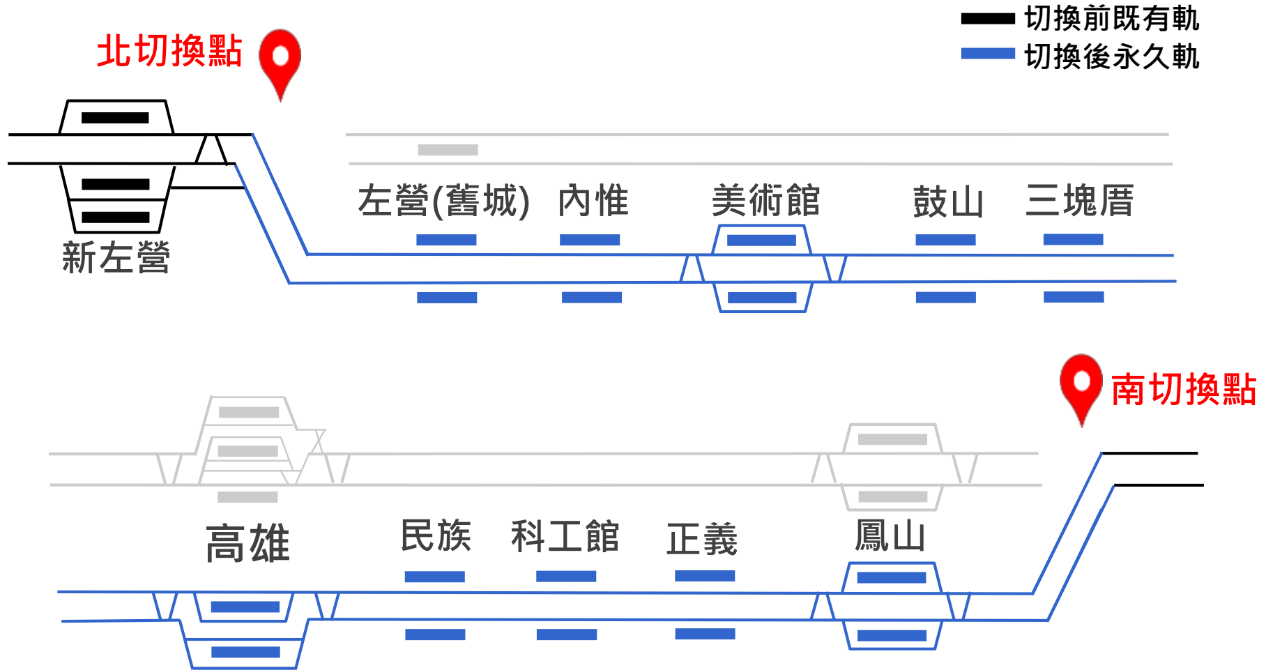
切換示意圖
