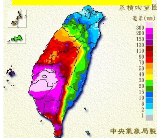
8月24日雨量圖
