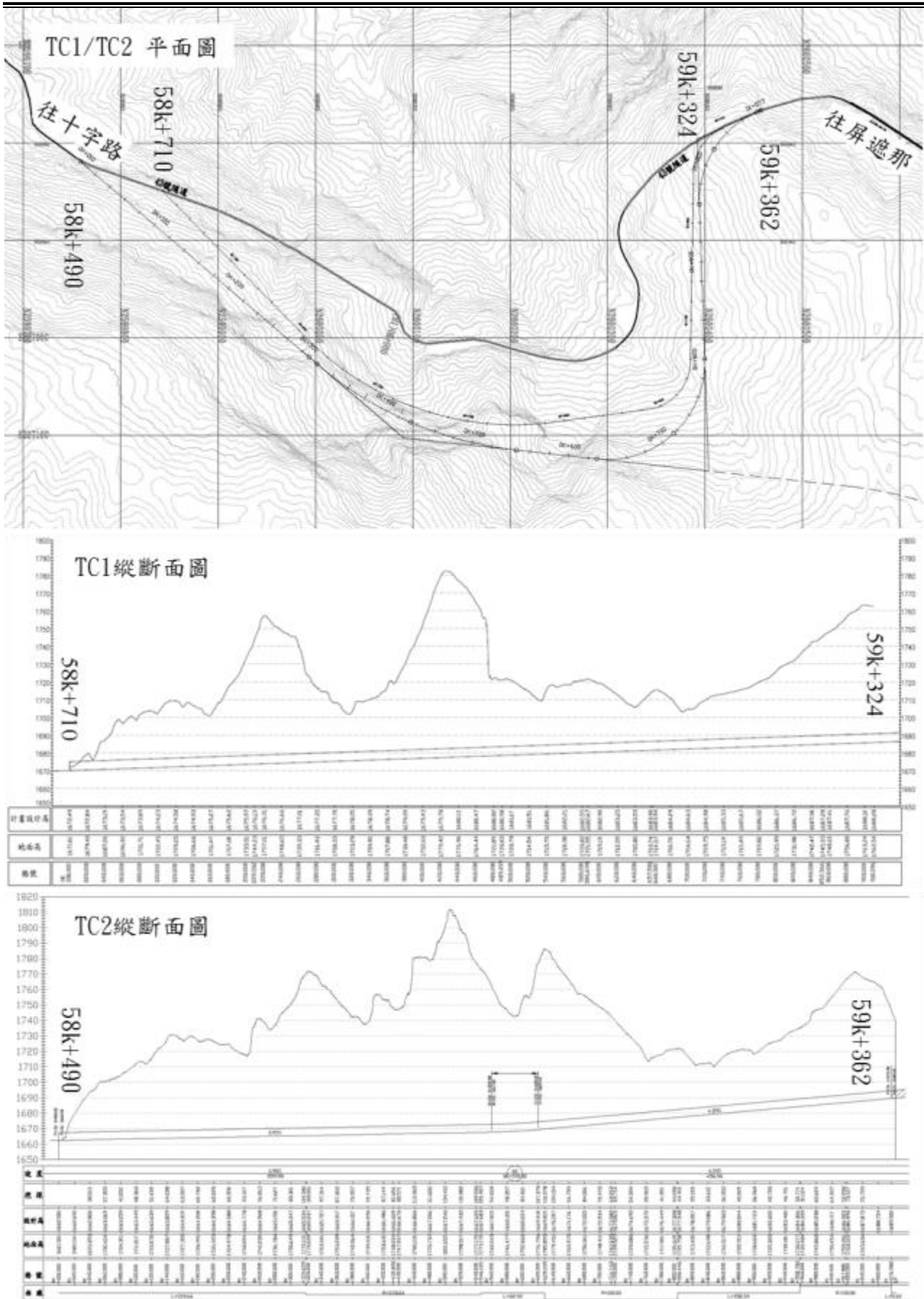
圖 8-1-4 方案 TC1&TC2 路線平縱斷面圖
