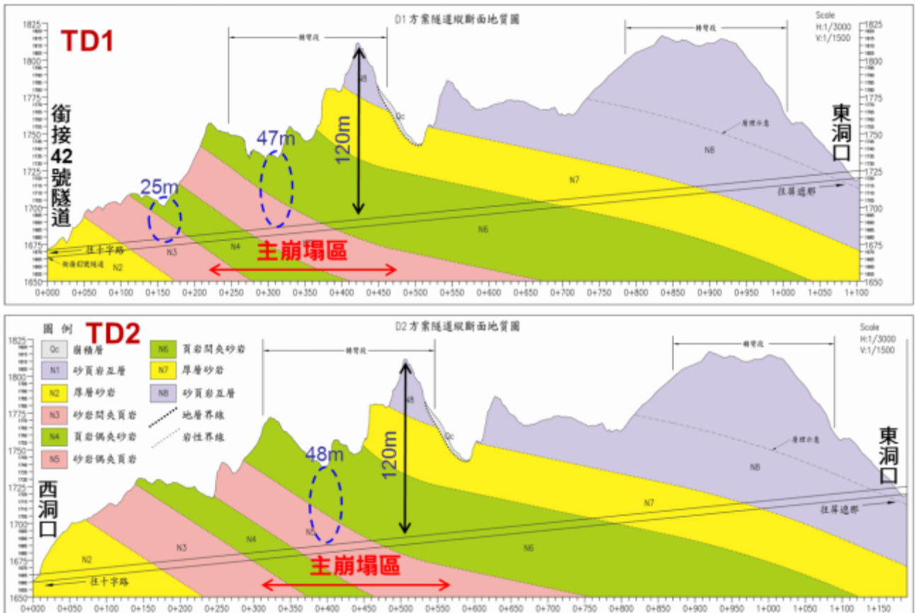
圖 8-1-8 方案 TD1&TD2 路線地質縱斷面圖
