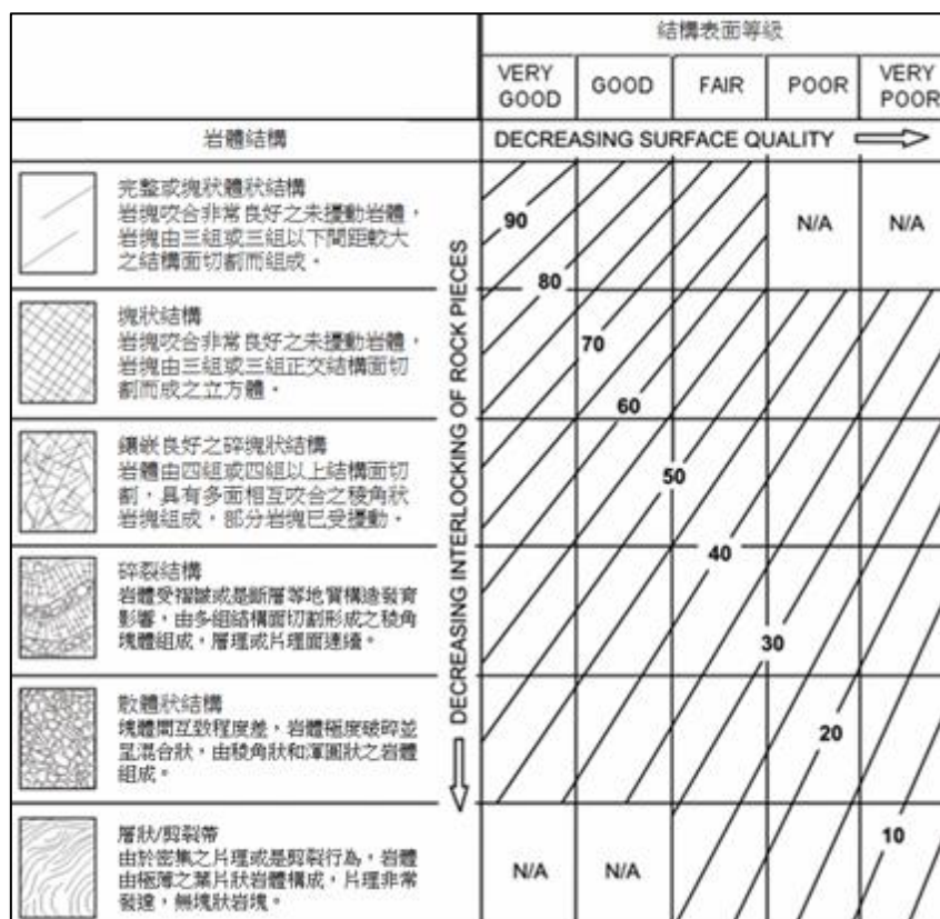
圖 3-2-7 地質強度指數(GSI)建議圖
