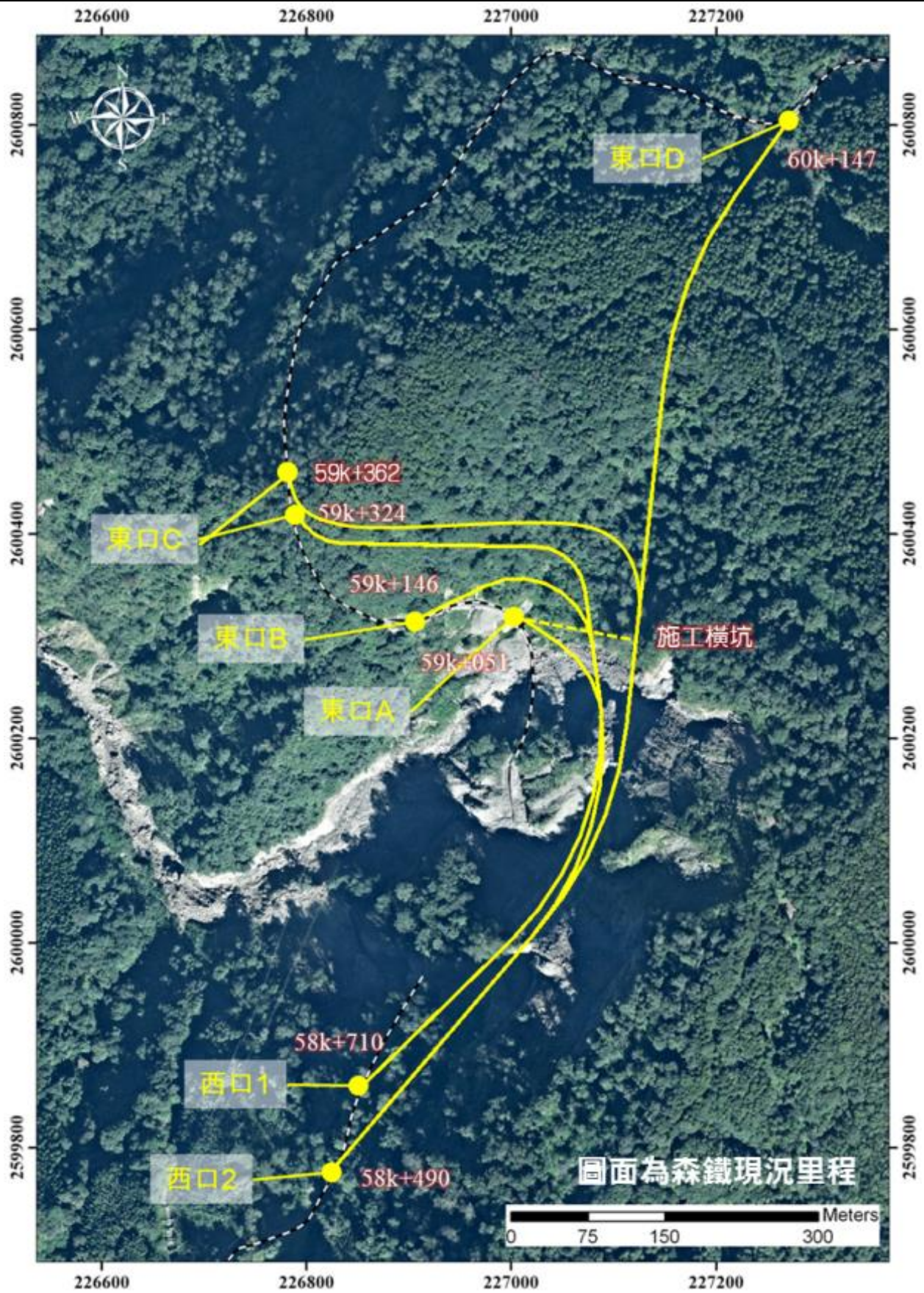
圖 8-1-3 可行隧道路線平面圖
