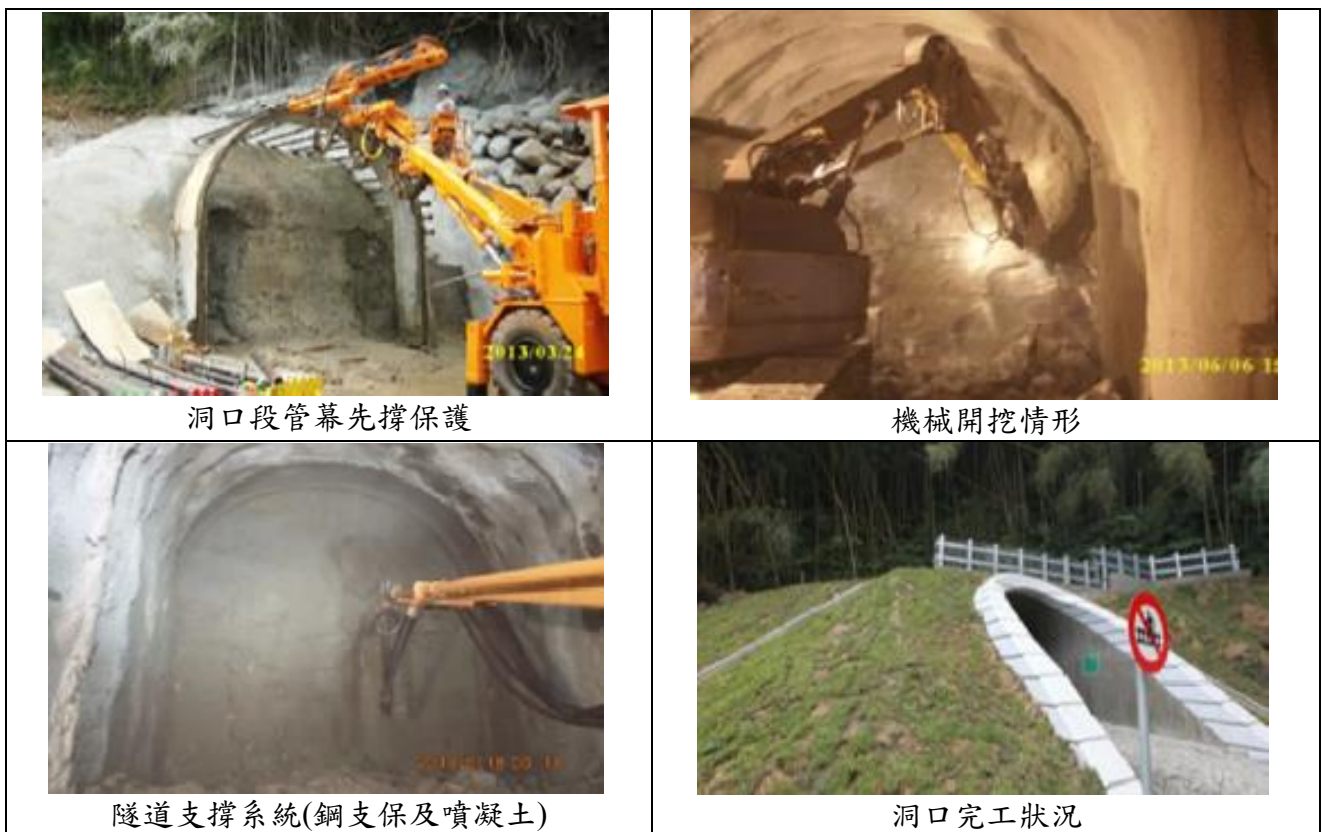
圖 3-2-6 隧道施工狀況案例圖
