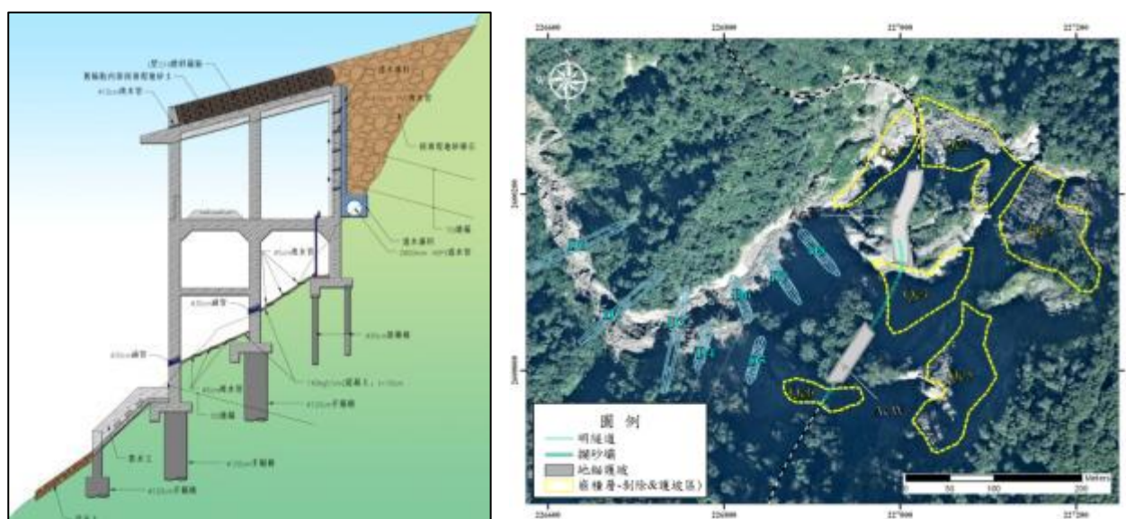
圖 8-1-1 明隧道配合水保設復建標準斷面及平面圖
