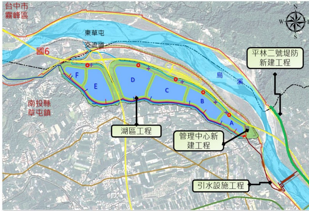
圖 1-2 本計畫工程佈置圖
