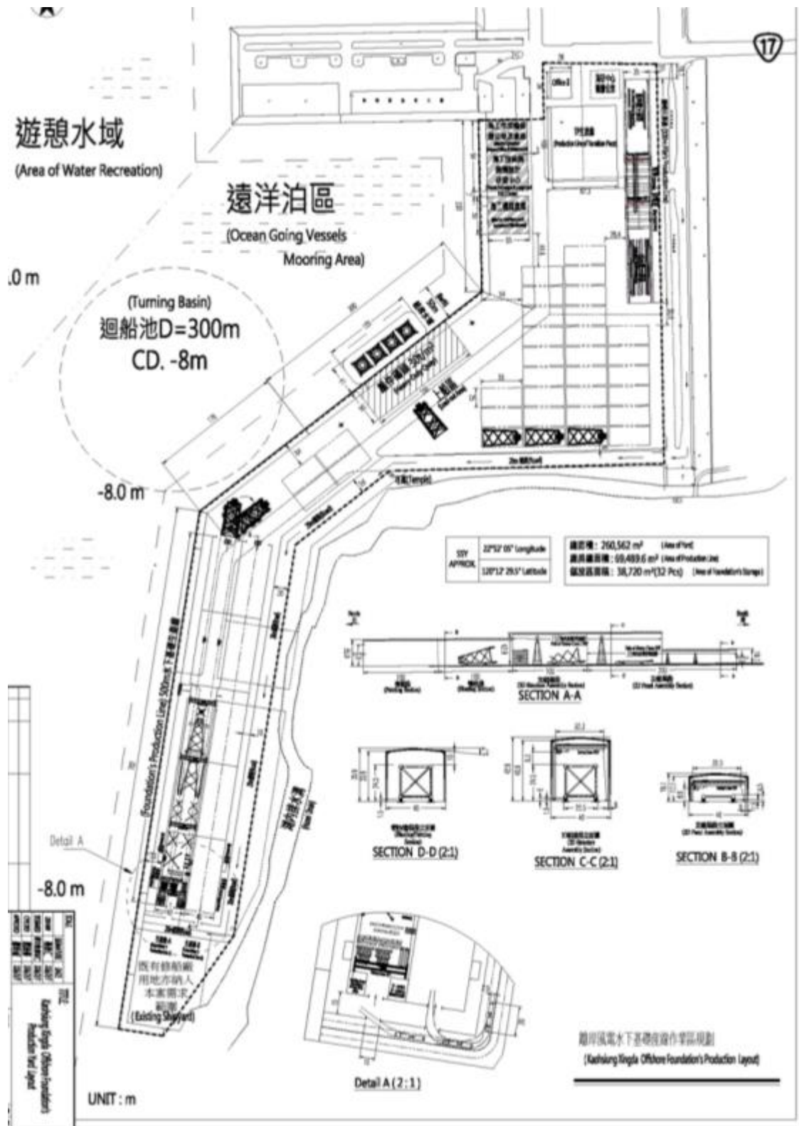
圖 4-3 海洋工程區規劃圖
