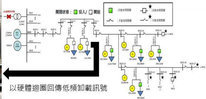
區域電網架構(台電雲林XG25饋線)
