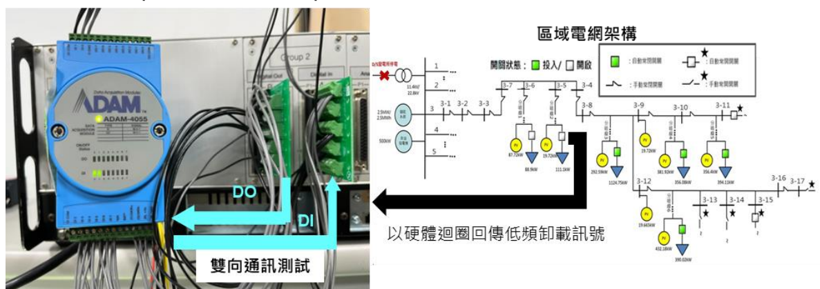
圖 67、硬體迴圈架構
