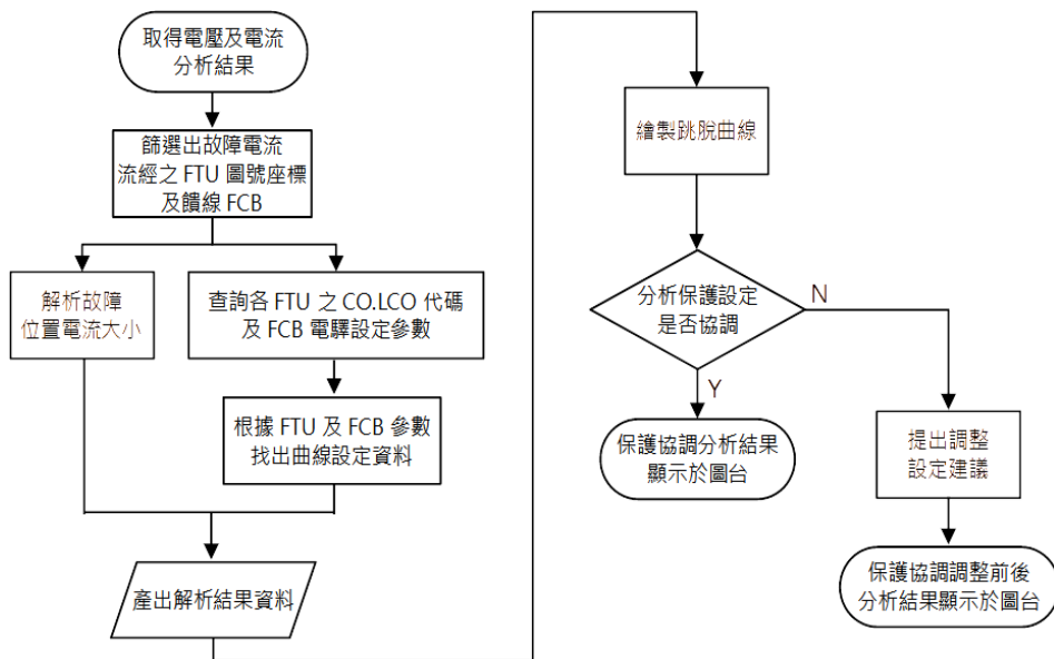
圖 47、適應性饋線架構之保護協調策略流程圖
