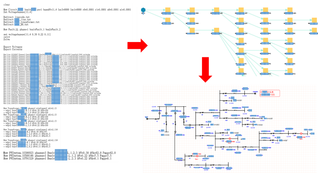
圖 48、撰寫程式，以圖形化呈現饋線架構，並建立饋線模型
