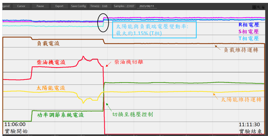
(b) 功率調節系統與多電源併聯基載補償實測
