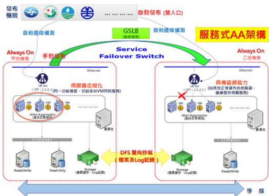
圖 25 災害訊息廣播服務平臺 A-A 架構圖
